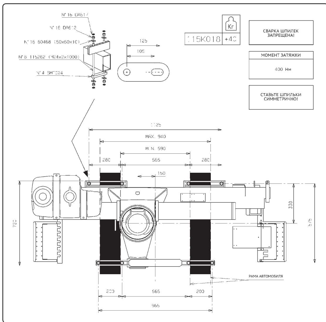
Рисунок 5 Монтажные размеры основания КМУ (п. 2.4.3)
